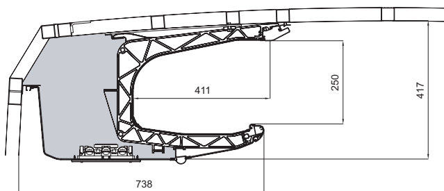
AREA SEZIONE PASSAGGIO ARIA PORTABAGAGLI: 87162 mm 2 - 0.09 m 2 AREA SECTION CHANNEL AIR PASSAGE: 87162 mm 2 - 0.09 m 2
