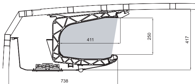
AREA SEZIONE VANO PORTABAGAGLI: 89914 mm 2 - 0.09 m 2 AREA SECTION BOOT: 89914 mm 2 - 0.09 m 2
